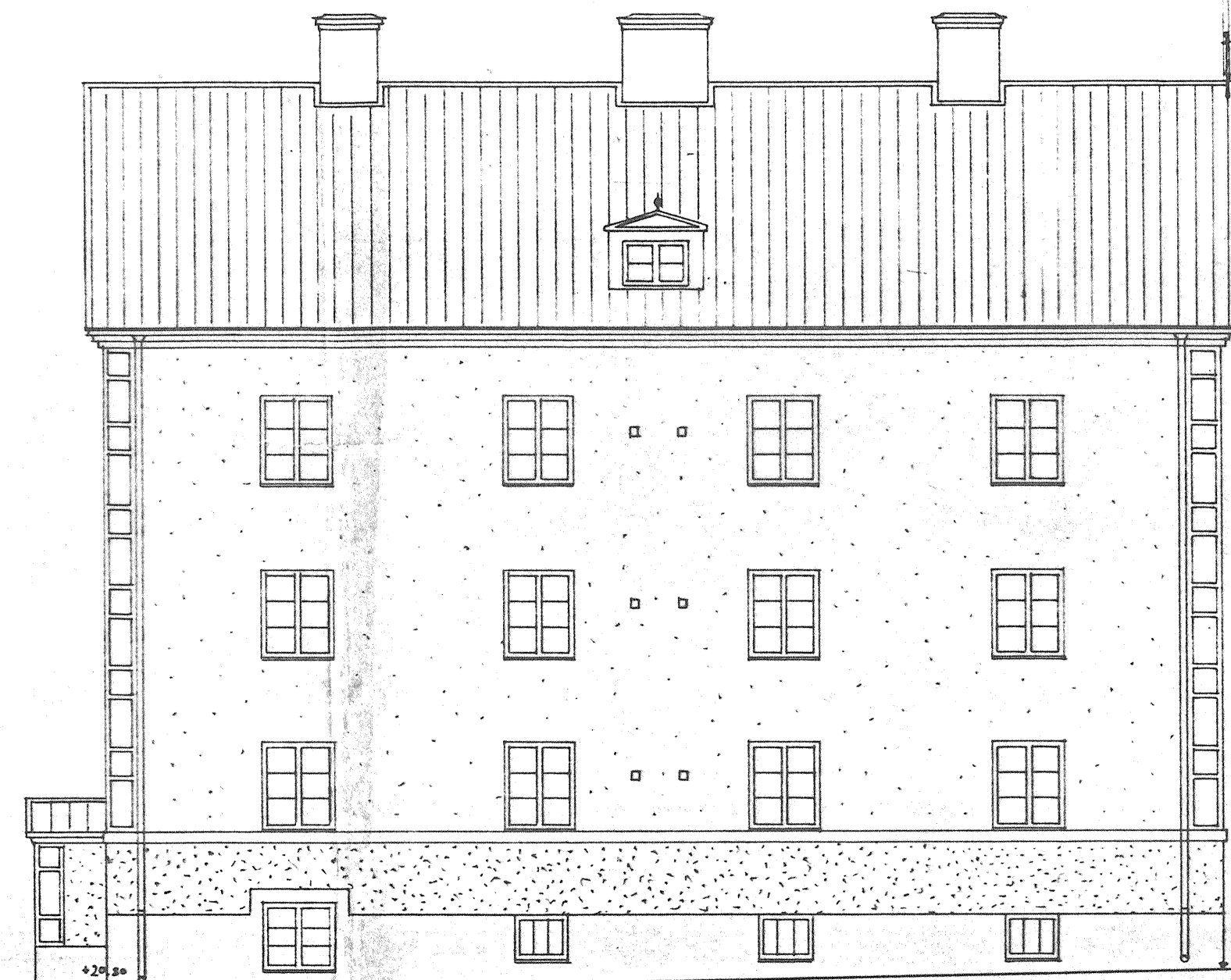
FASAD MOT SUNDELIUSGATAN.
